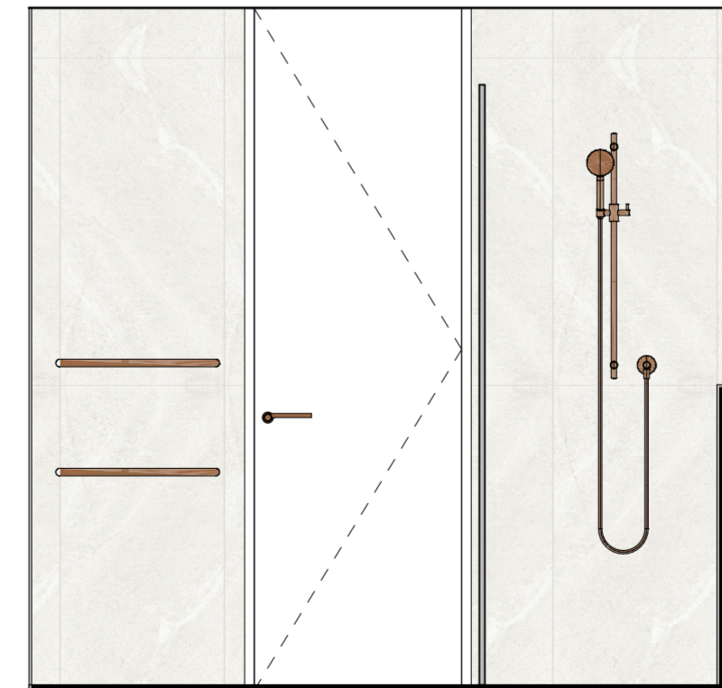
04 Bathroom Elevation SCALE: 1:25
