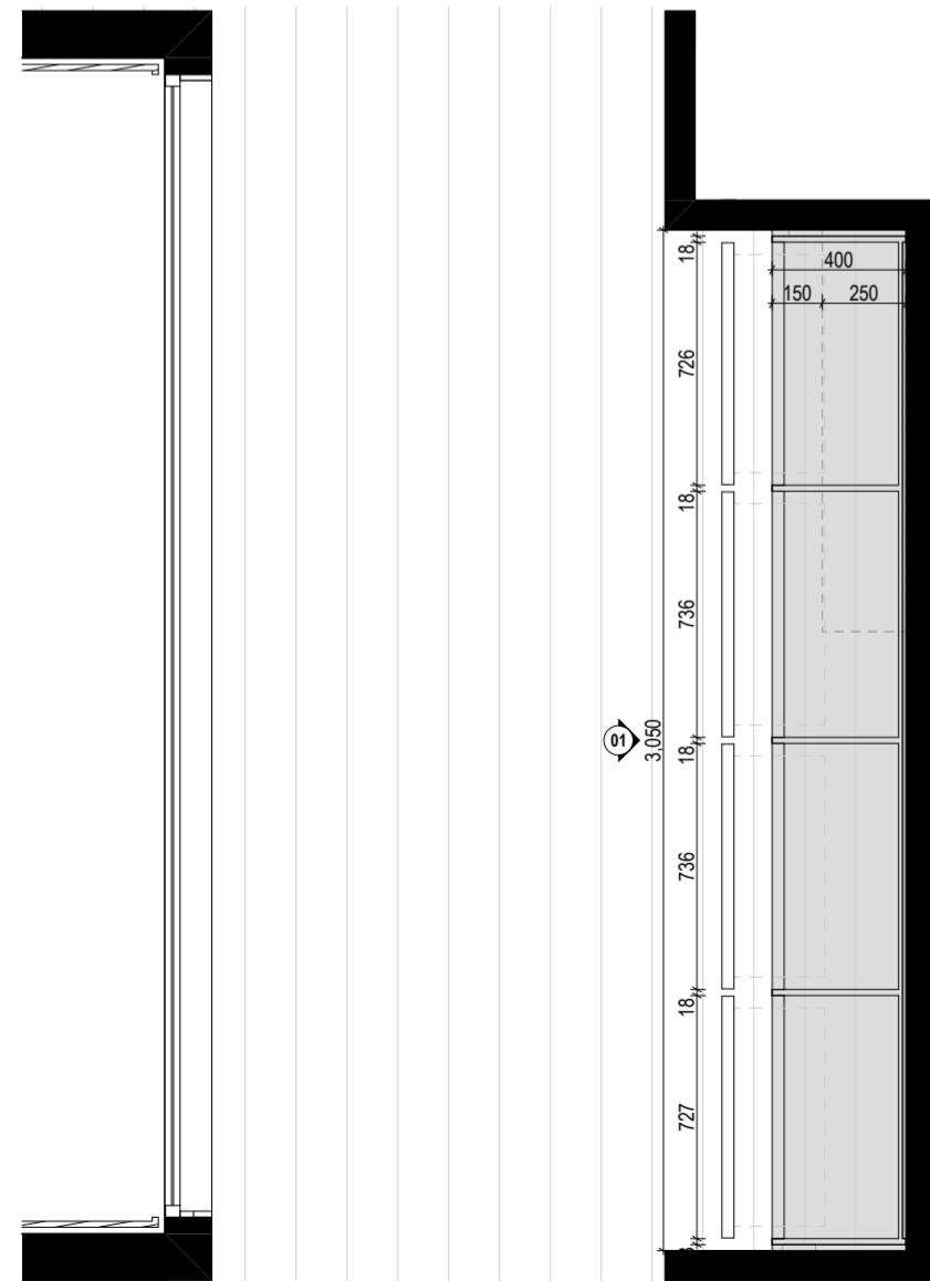
Hallway Plan SCALE: 1:25
