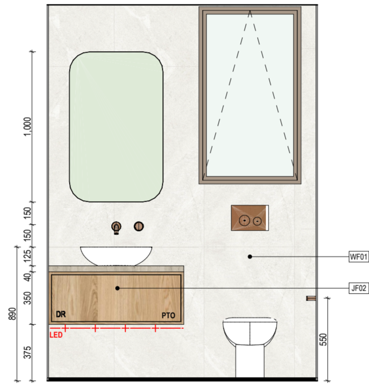
01 Ensuite 2 Elevation
