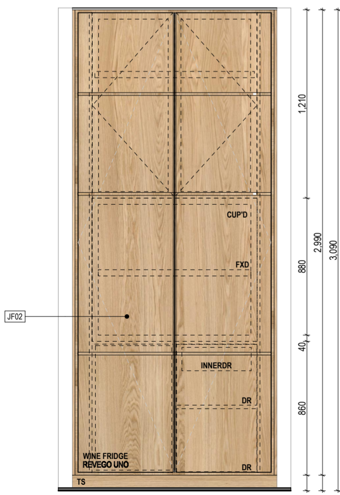
06 Breakfast Bar Elevation SCALE: 1:25
