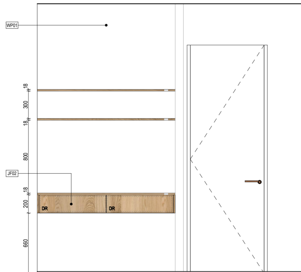
01 Bedroom 01 Elevation SCALE: 1:25
