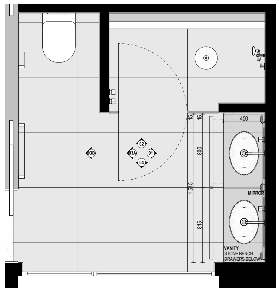
Ensuite Plan SCALE: 1:25
