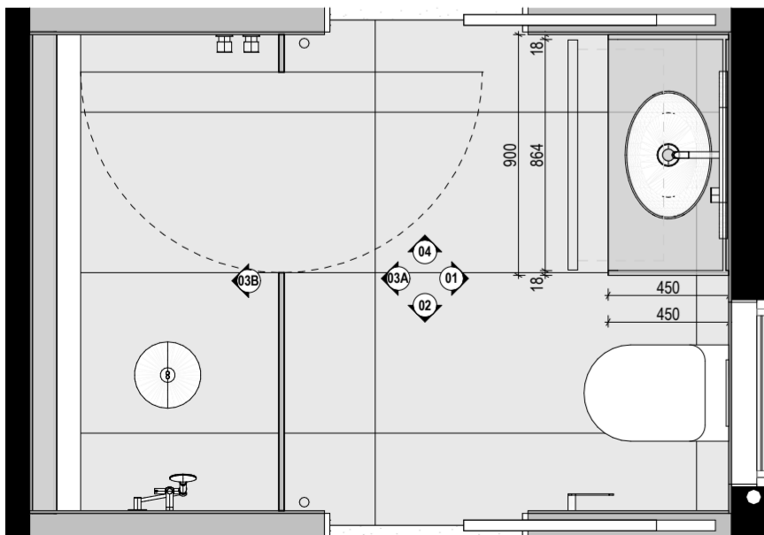
Ensuite 02 Plan
