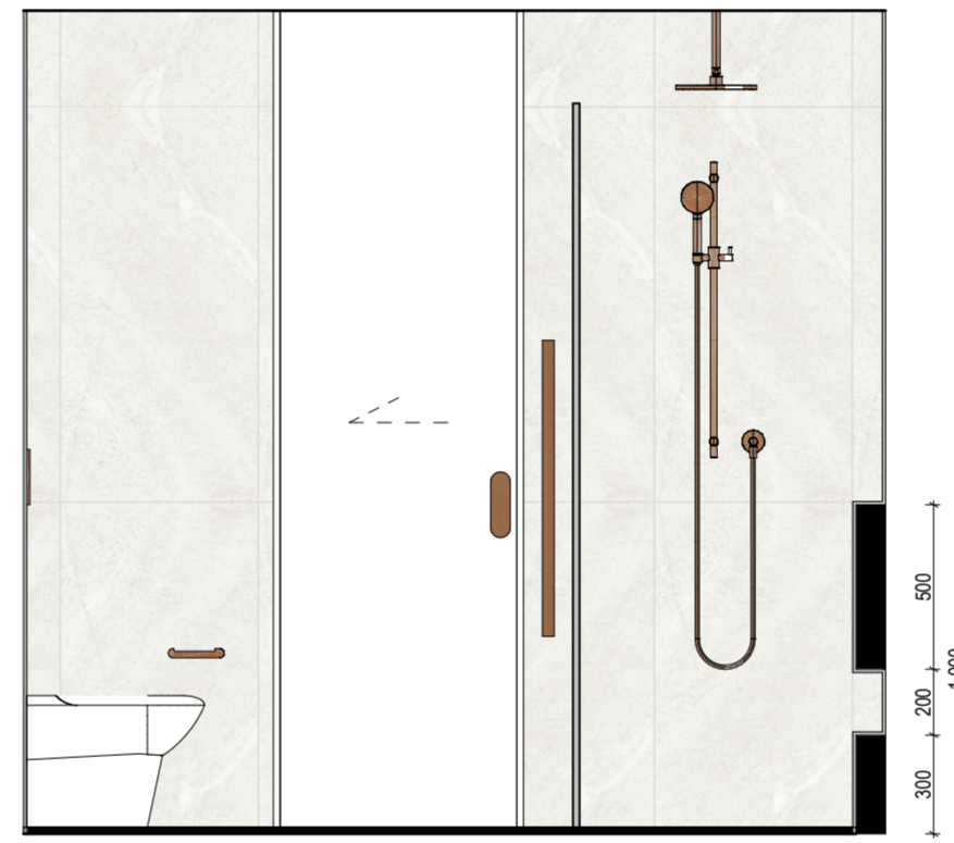
02 Ensuite 2 Elevation
