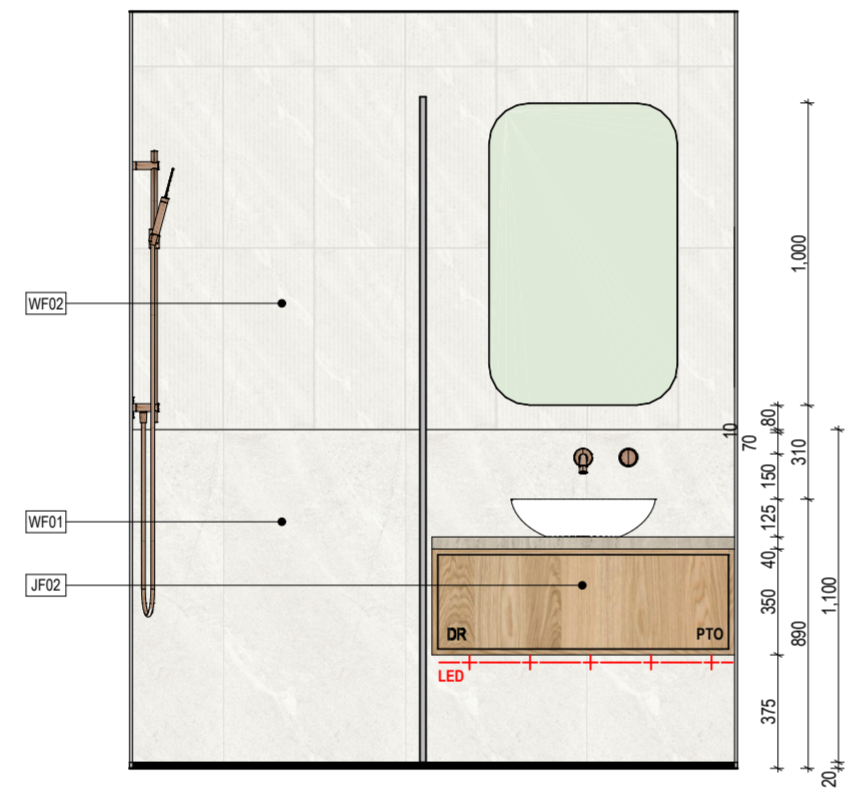
01 Bathroom Elevation SCALE: 1:25
