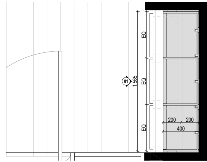
Entry Plan SCALE: 1:25
