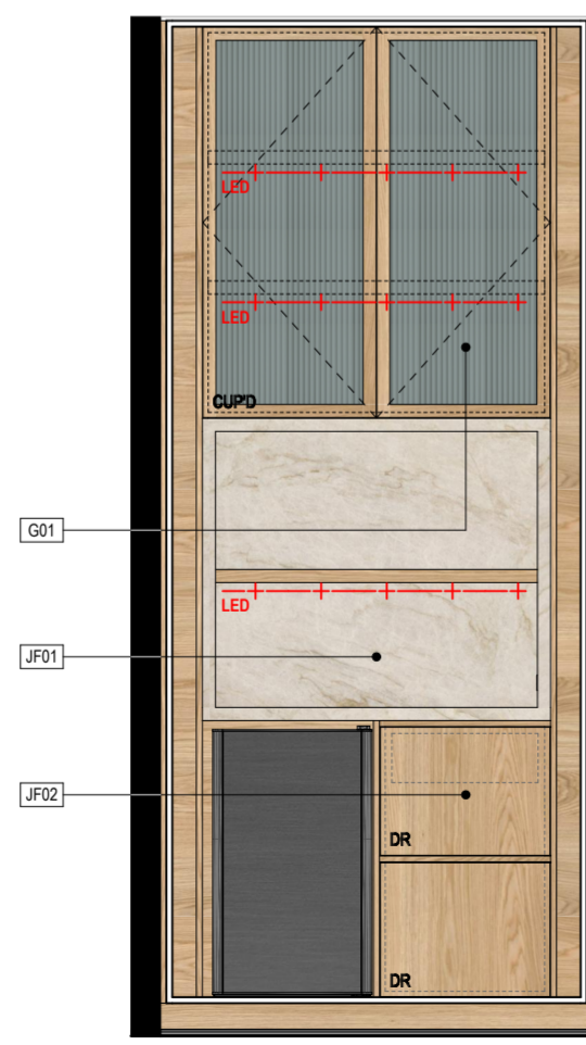
07 Breakfast Bar Internal SCALE: 1:25
