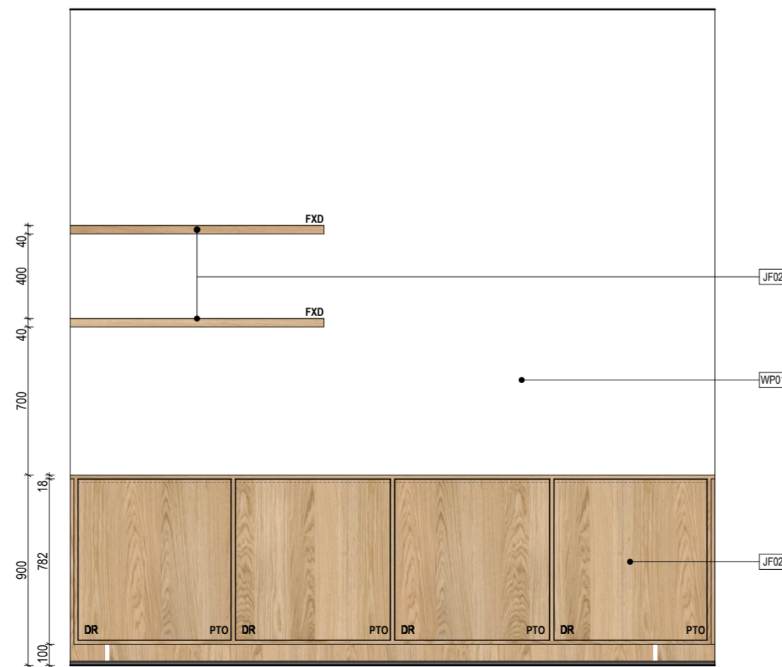
01 Hallway Elevation SCALE: 1:25
