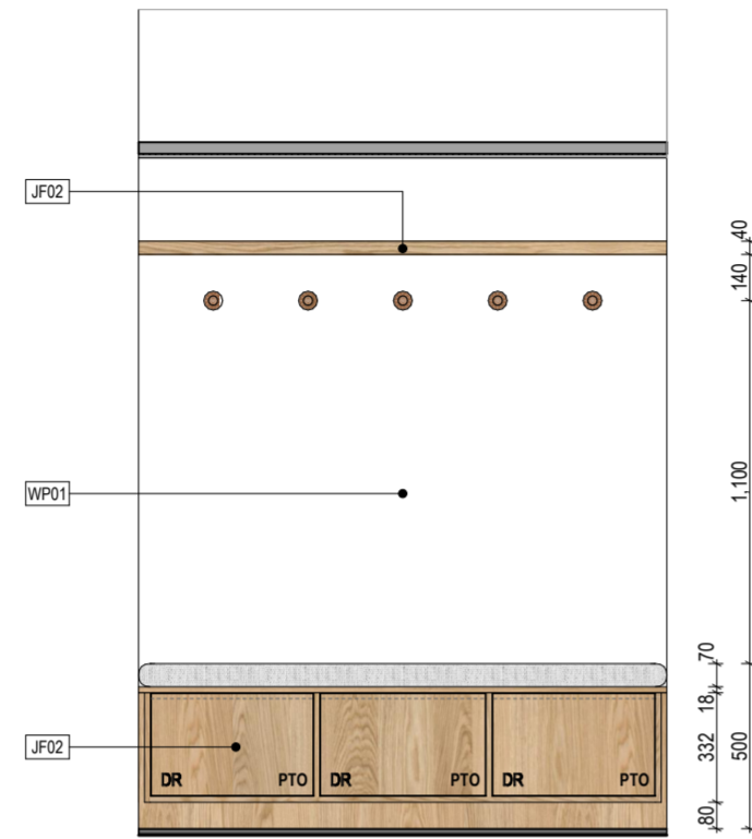
01 Entry Elevation SCALE: 1:25
