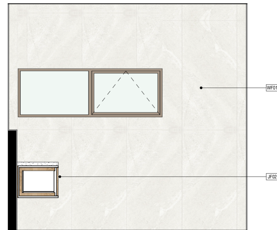
02 Bathroom Elevation SCALE: 1:25
