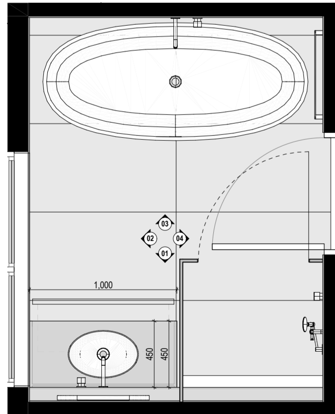
Bathroom Plan SCALE: 1:25
