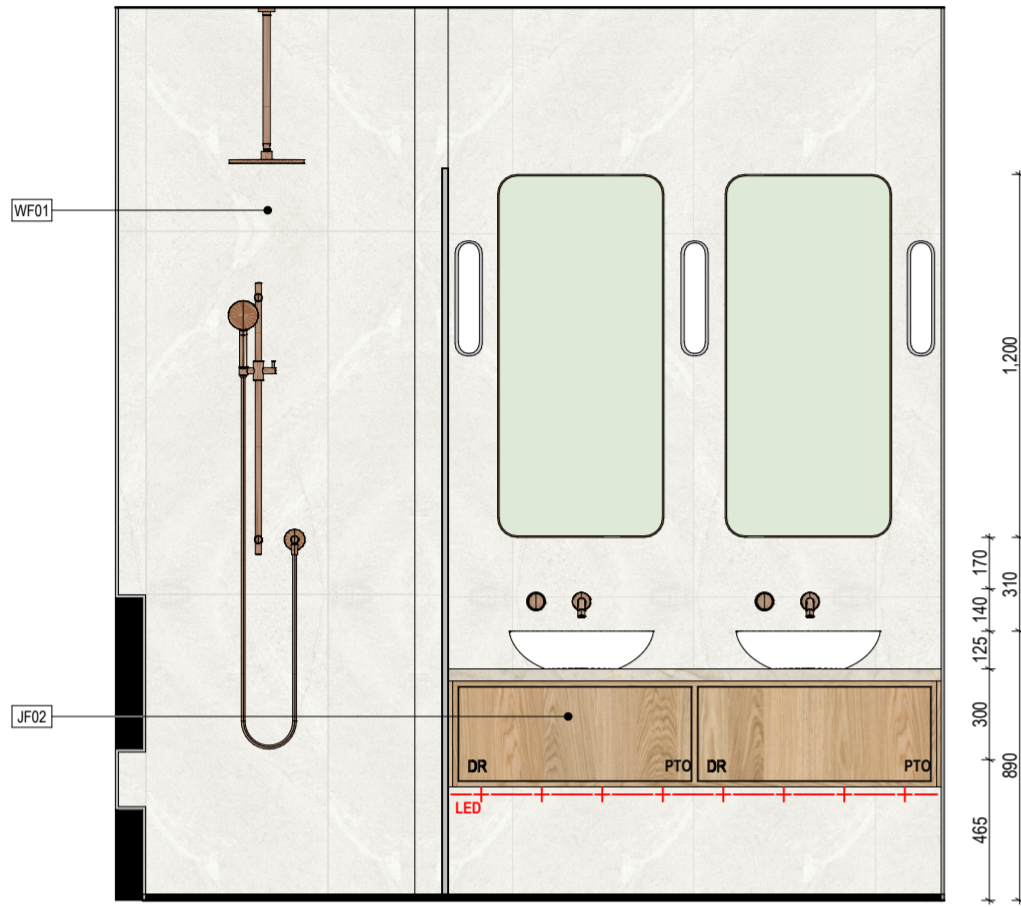
01 Ensuite Elevation SCALE: 1:25
