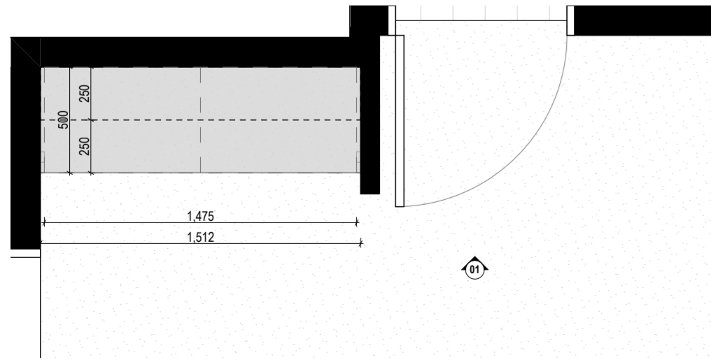
Bedroom 01 Plan SCALE: 1:25
